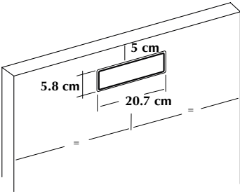
Touch handle with profile WY1 maniglia Touch con profilo WY1 poignée Touch avec profil WY1 tirador Touch con perfil WY1
