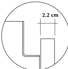
door thickness . spessore anta épaisseur de la porte . espesor de puerta
